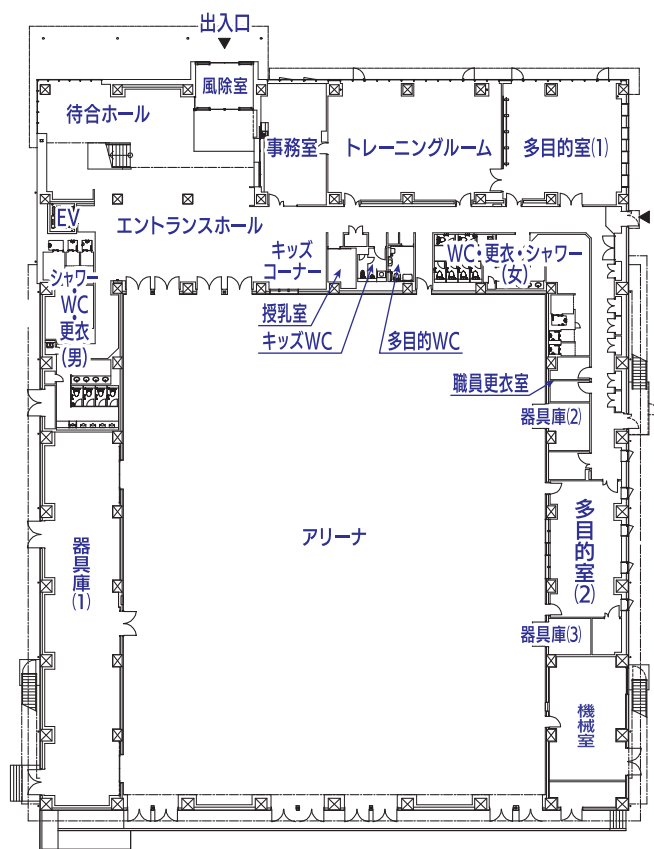
1階平面図
